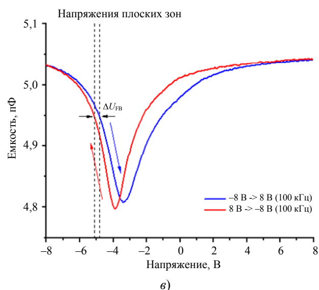
Рис. 3. Вольт-фарадные характеристики трёх типов МДП-структур при T = 78\text{ К} : (а) \text{Ni}/\text{Al}_2\text{O}_3/\text{HgCdTe} ; (б) \text{Ni}/\text{SiO}_x(30\text{ нм})/\text{Al}_2\text{O}_3/\text{HgCdTe} и (в) \text{Ni}/\text{SiO}_x(350\text{ нм})/\text{Al}_2\text{O}_3/\text{HgCdTe}
