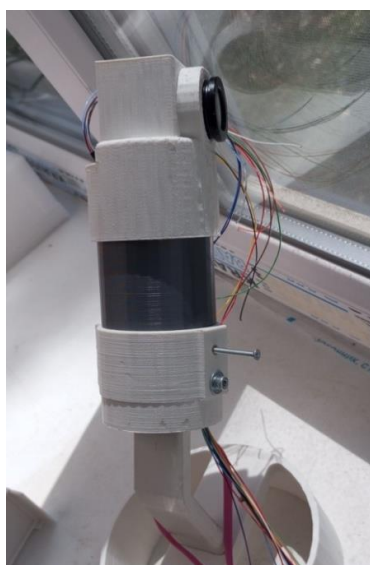
Рис. 7. Модель и внешний вид разрабатываемой системы для определения атмосферной видимости в дневное время по изображениям Солнца
