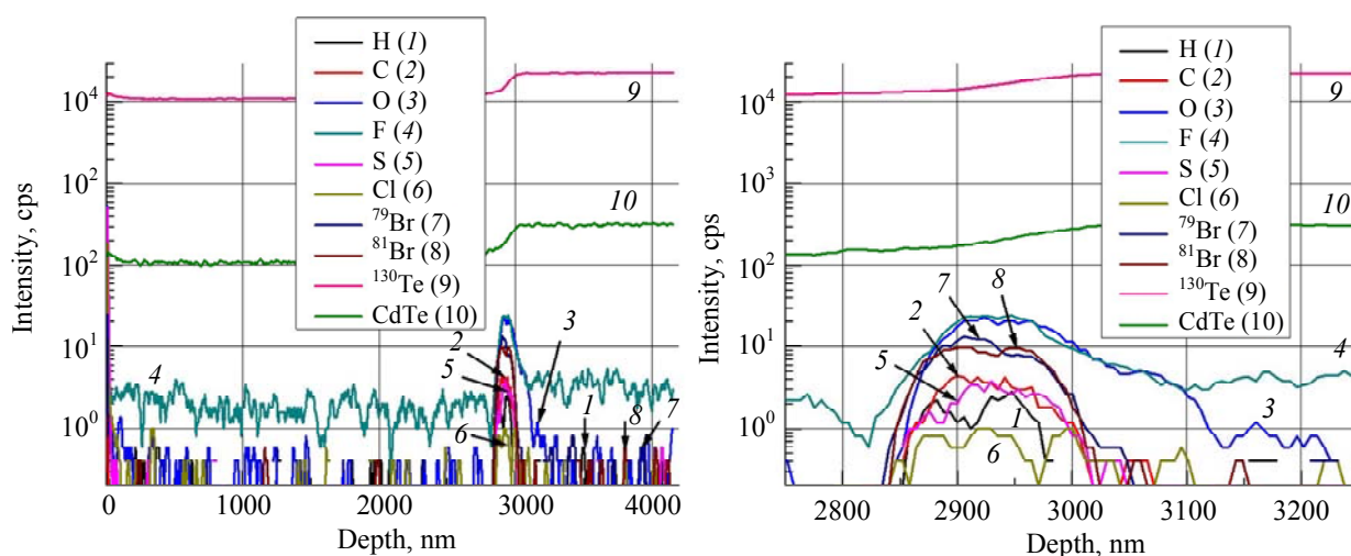
Рис. 2. ВИМС-профиль гетероструктуры Cd_{0,3}Hg_{0,7}Te/Cd_{0,96}Zn_{0,04}Te (211)В в отрицательных ионах. На рисунке справа более подробно показана область гетерограницы слой-подложка
