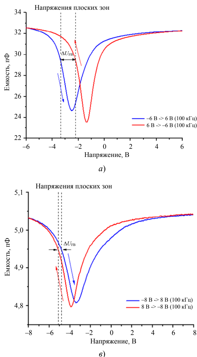
Рис. 3. Вольт-фарадные характеристики трёх типов МДП-структур при T = 78\text{ К} : (а) \text{Ni}/\text{Al}_2\text{O}_3/\text{HgCdTe} ; (б) \text{Ni}/\text{SiO}_x(30\text{ нм})/\text{Al}_2\text{O}_3/\text{HgCdTe} и (в) \text{Ni}/\text{SiO}_x(350\text{ нм})/\text{Al}_2\text{O}_3/\text{HgCdTe}
