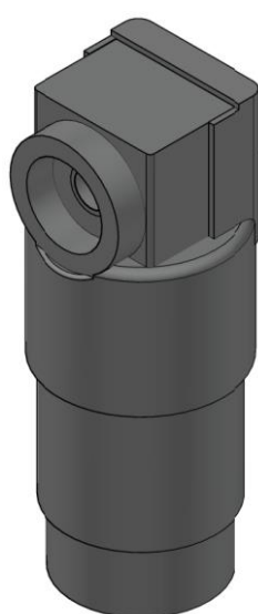
Рис. 7. Модель и внешний вид разрабатываемой системы для определения атмосферной видимости в дневное время по изображениям Солнца
