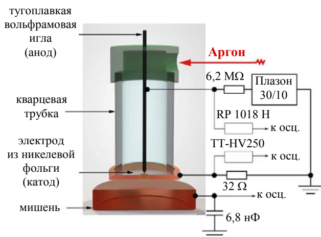
Рис. 1. Экспериментальная установка
