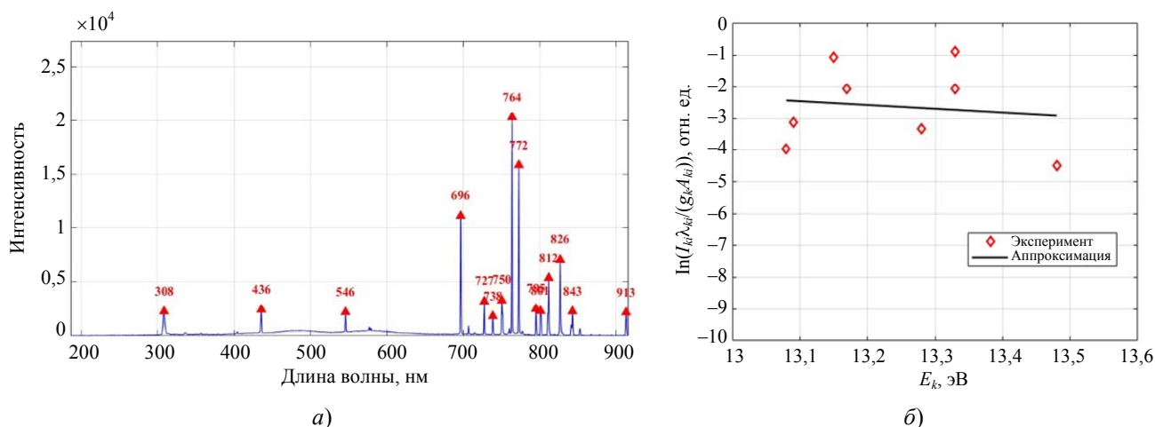
Рис. 4. а) – спектр оптического излучения плазмы в аргоне при подаче постоянного напряжения; б) – график Больцмана для перехода линии Ar I (4s-4p)
