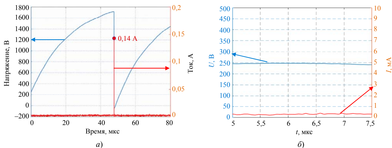
Рис. 2. Два режима разряда при постоянном напряжении: а) – самоподдерживающийся, б) – тлеющий
