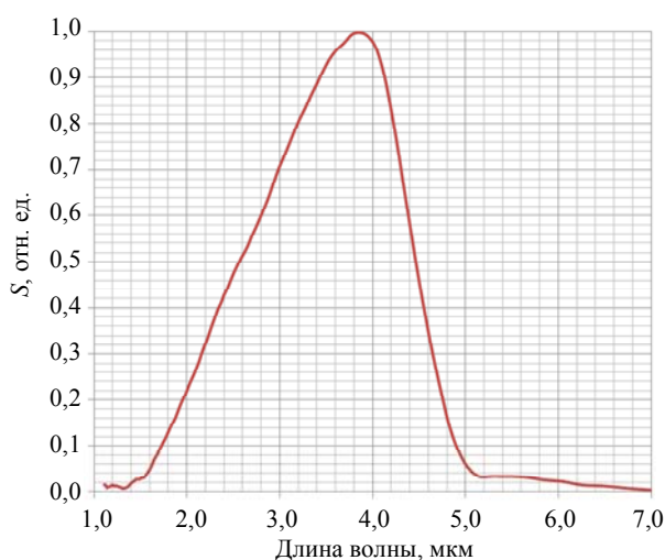
а) МФЧЭ-01 со сверхрешеткой в качестве барьера
