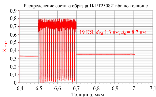
а) n\text{Вn} -гетероструктура на основе ГЭС КРТ МЛЭ со сверхрешеткой в качестве барьера
