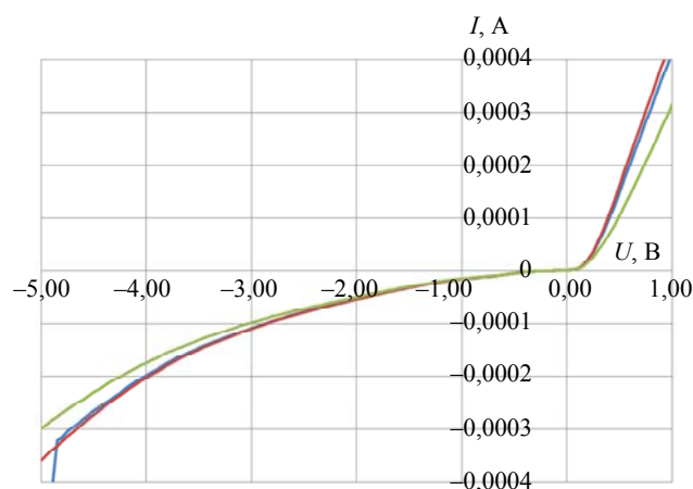
а) МФЧЭ-01 со сверхрешеткой в качестве барьера
