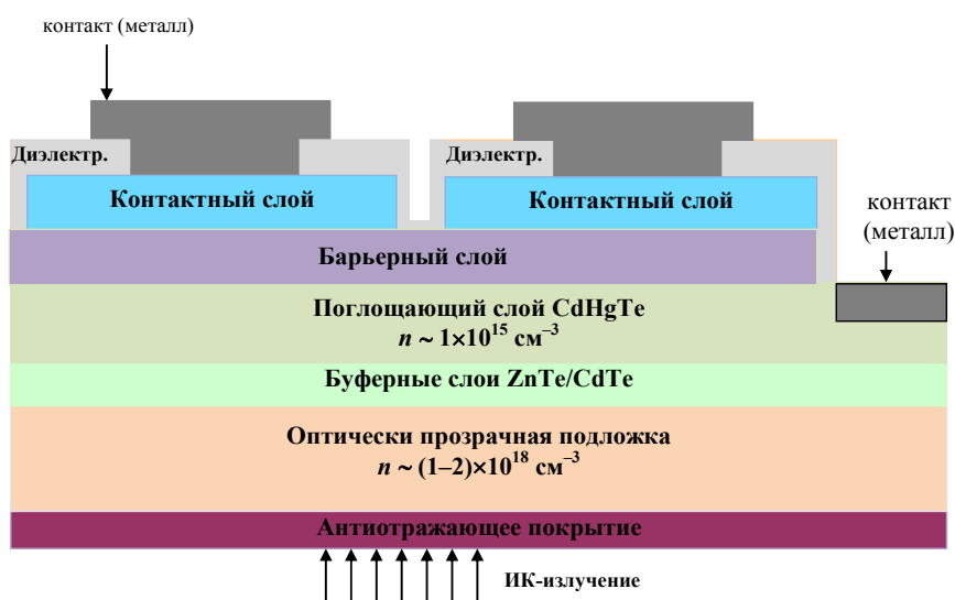
Рис. 5. Схематичное представление фрагмента МФЧЭ на основе CdHgTe
