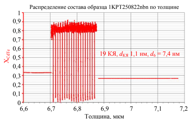
б) n\text{Вn} -гетероструктура на основе ГЭС КРТ МЛЭ со сверхрешеткой в качестве барьера
