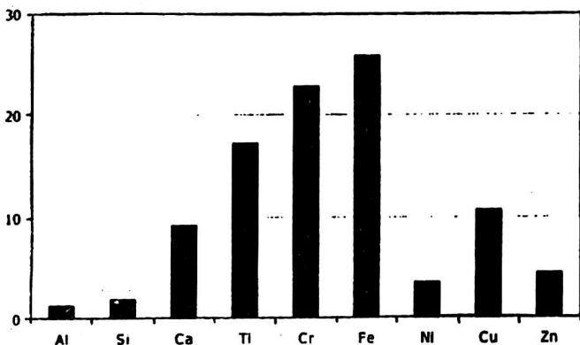
Рис. 11. Средний по результатам 5 опытов процент атомов "чужих" элементов при нагрузке из циркония
