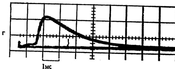
Рис. 2. Типичные осциллограммы: а — напряжения; б — тока в нагрузке; в — сигнала с фотодиода; г — сигнала с ФЭУ-35, стоящего за интерференционным фильтром \lambda = 432 \text{ нм}
