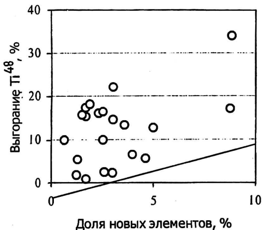
Рис. 10. Корреляция уменьшения доли Ti^{48} и увеличения доли "чужих" элементов (проценты по весу)
