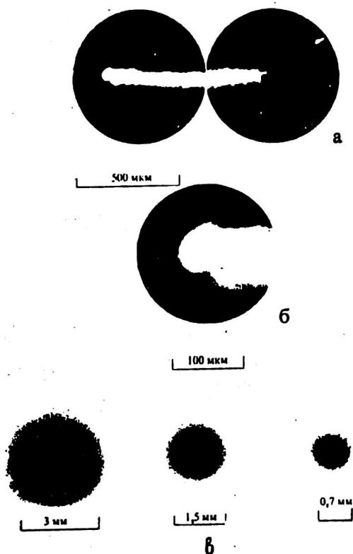
Рис. 16. След типа “кометы” (а); увеличенный фрагмент “головы кометы” (б); след “слоеном” (в)
