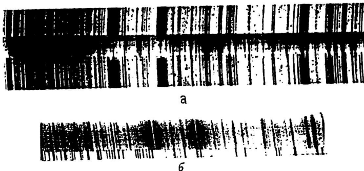
Рис. 6. Фрагмент спектра излучения плазмы, снятый спектрометром ИСП-51 (верхний и нижний спектры опорные — Si и Zn) — а; фрагмент спектра излучения плазмы (вверху) и опорного спектра железа (внизу) в диапазоне длин волн 3800—4100 Å, снятый спектрометром СТЭ-1 — б
