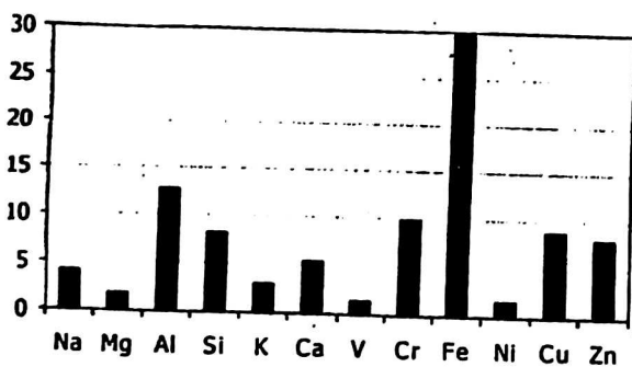
Рис. 9. Средний по результатам 24 опытов (№ 169—240) процент атомов “чужих” элементов при нагрузке из титана
