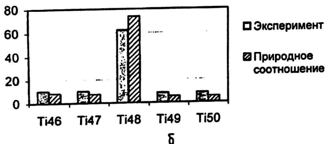
Изотопный состав Ti , %
