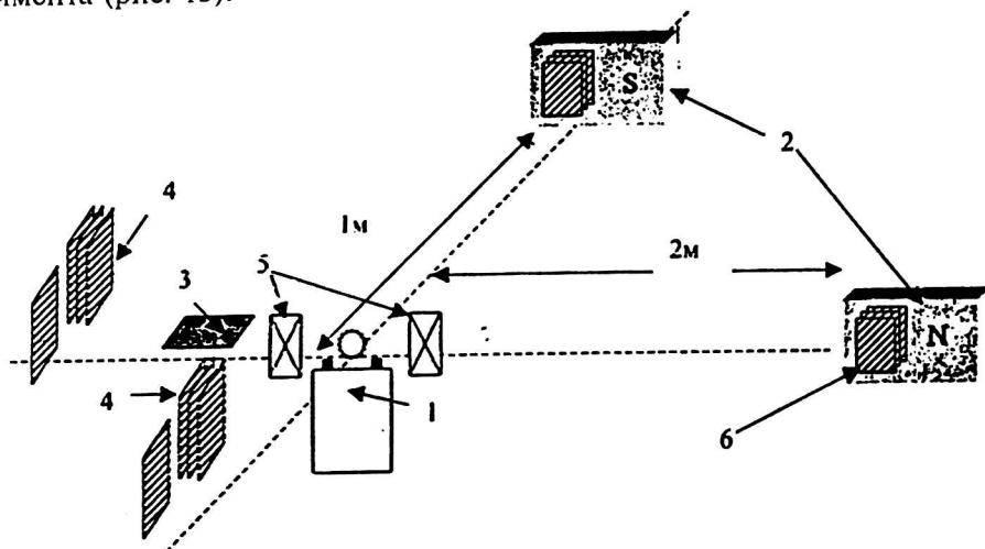
Рис. 13. Схема расположения фотодетекторов:
