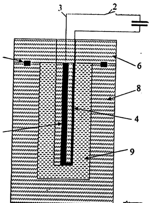
Рис. 1. Схема эксперимента: 1 — конденсаторная батарея; 2 — разрядник; 3 — кабель; 4 — фольга; 5 — электрод; 6 — полиэтиленовая крышка; 7 — уплотнение; 8 — взрывная камера; 9 — дистиллированная вода
