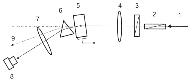
Рис. 2. Оптическая схема экспериментальной установки.
