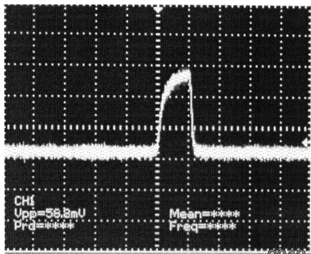
Рис. 3. Оптический сигнал, регистрируемый фотоприемником.
