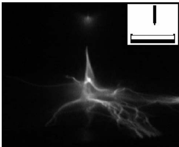
Рис. 1. Фотография иллюстрирующая эволюцию горения отрицательной короны с диэлектрическим барьером. Диэлектрический барьер – полимерная пленка, толщина d = 60 мкм.
