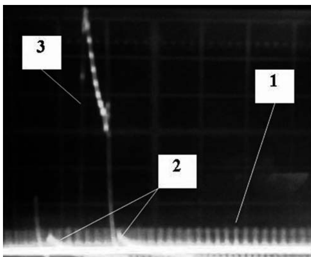
Рис. 2. Осциллограммы импульсов тока: 1 – отрицательной короны с диэлектрическим барьером ( I = 184 мкА, T = 40 мкс); 2 – слабого поверхностного разряда ( I = 44 мкА, T = 1,2 мс); 3 – импульс тока стримерного разряда ( I = 1,4 мА, T = 0,3 мс).
