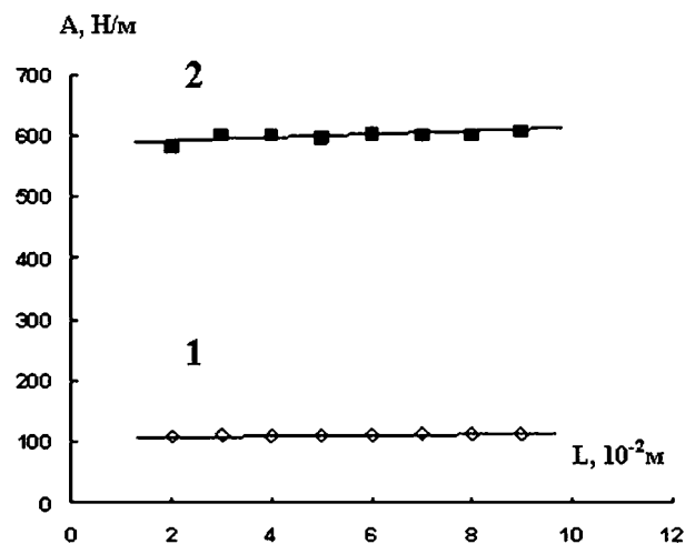
Рис. 3. Измерение сопротивления отслаивания A от исходной (1) и модифицированной (2) поверхности ПТФЭ.
