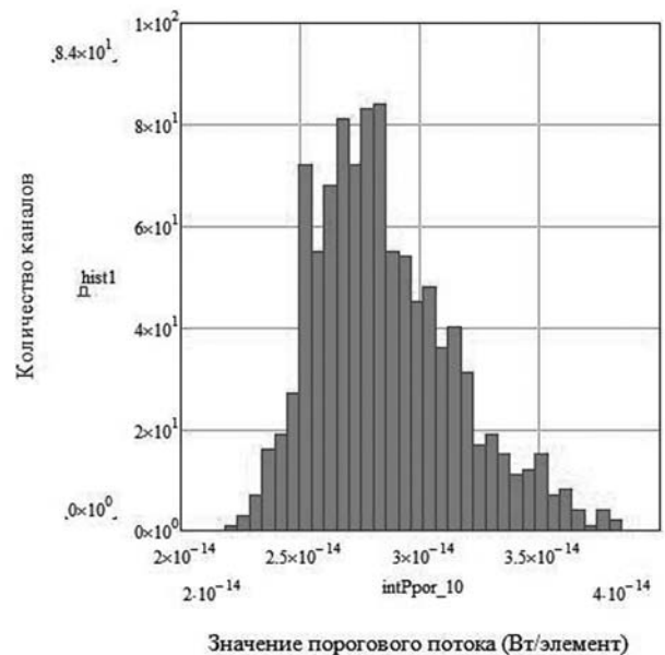
Рис. 5. Гистограмма значений порогового потока.
