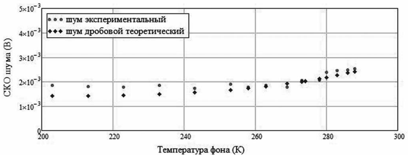
Рис. 4. Зависимости усредненного по каналам значения шума и теоретические расчеты дробового шума на выходе БИС считывания от температуры заслонки.
